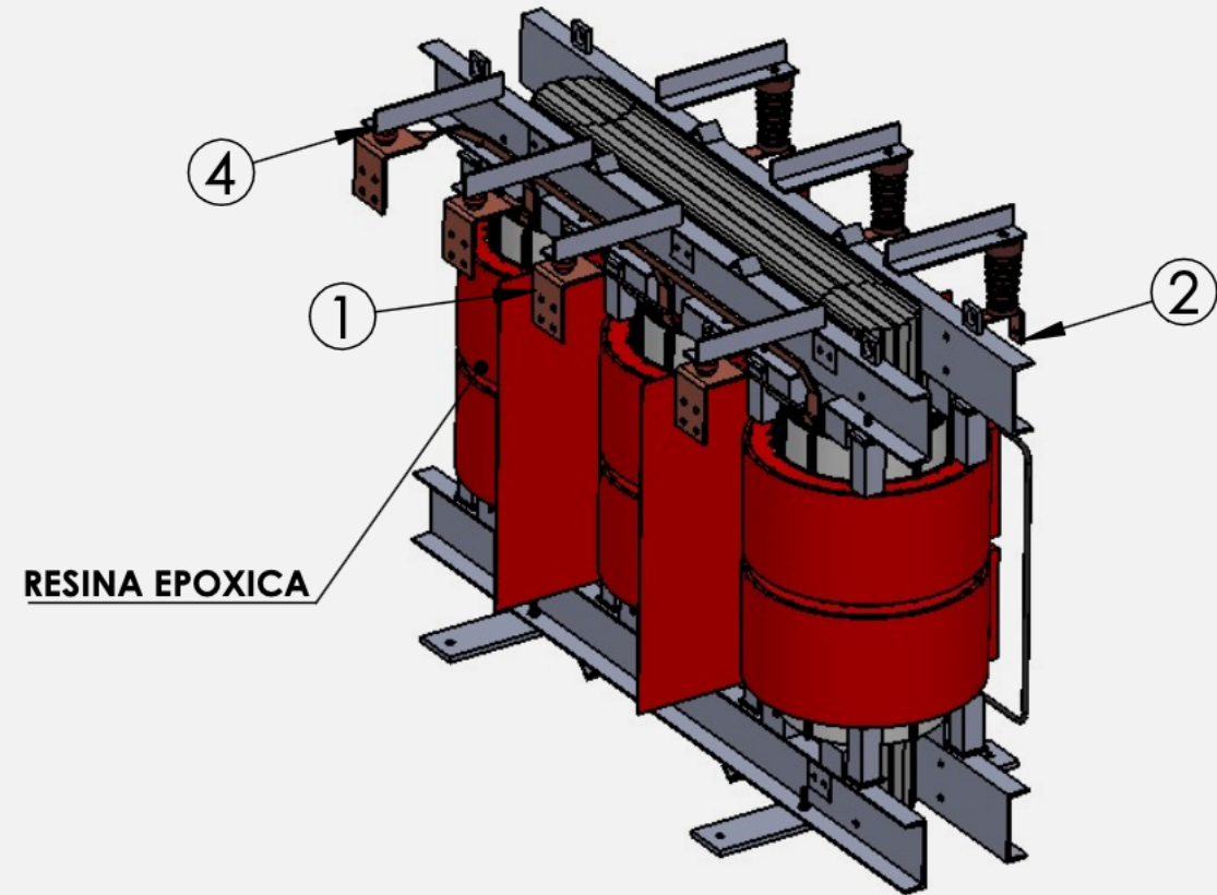
Vista isométrica interior
